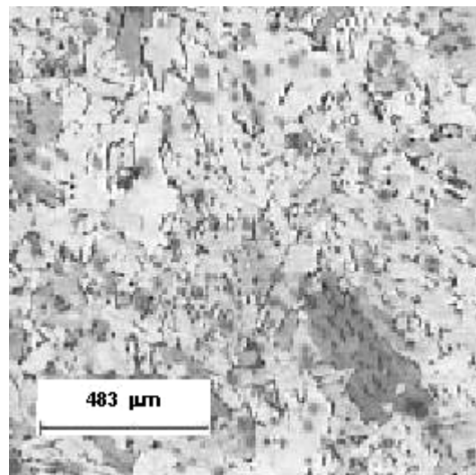
Figura 7. Microestrutura do centro da placa de aço microligado.
